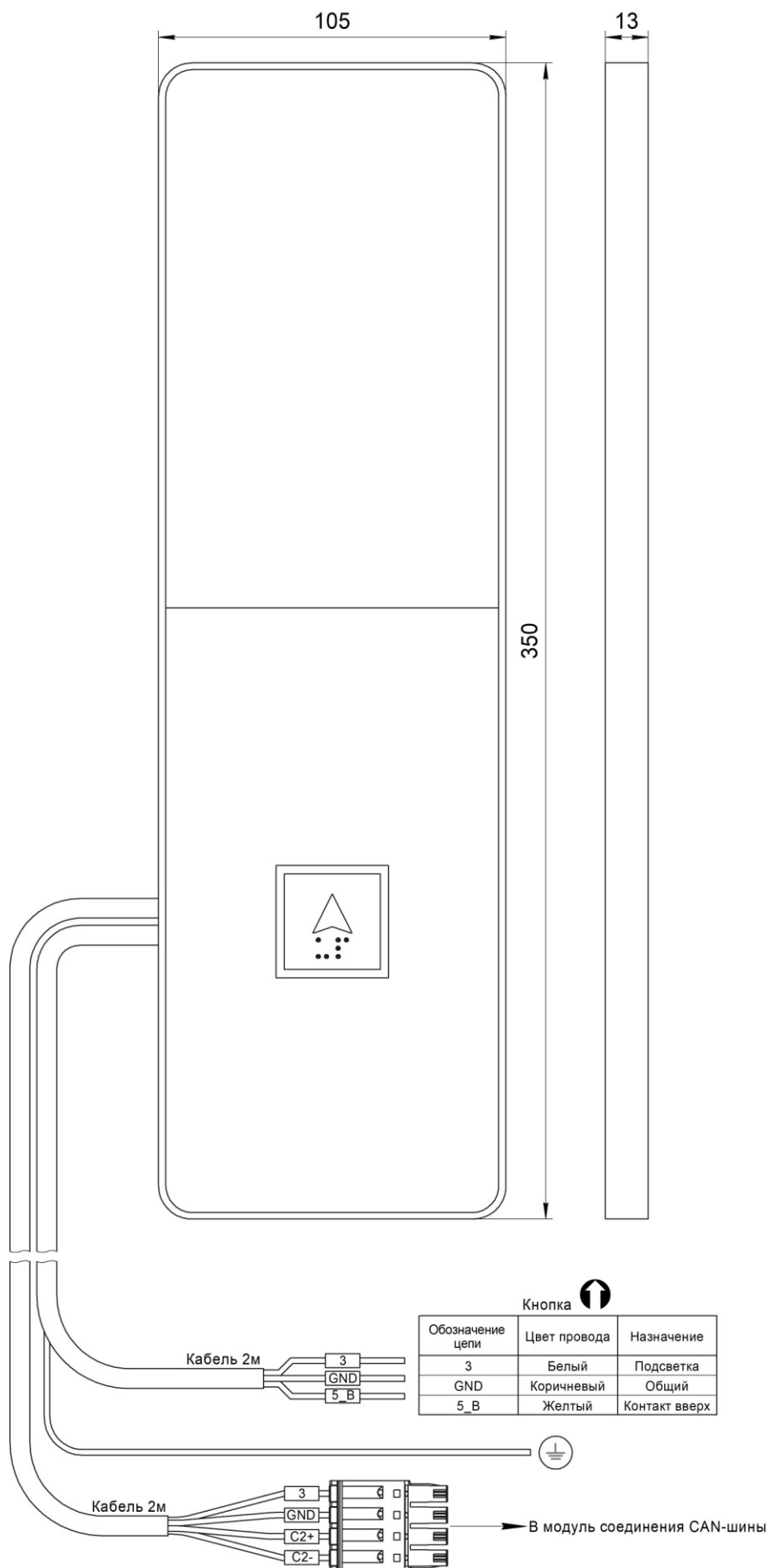
Рис.1 Внешний вид, габаритные и установочные размеры Вызывного поста МАЛАХИТ НШЕК.468381.085
